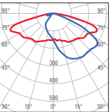
DE = Ottica stradale Classe M3-M4 larghezza carreggiata > altezza palo Road optic Class M3-M4 larghezza carreggiata > pole height
