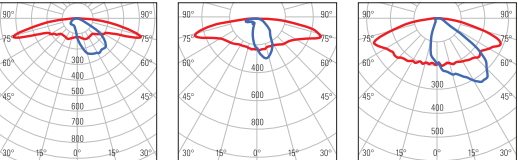
DA = Ottica stradale e ciclopeditonale estensiva Classe P - Type II/III (long) ad elevata interdistanza Extensive road and cycle-pedestrian optic Class P - Type II/III (long) for high pole spacing DB = Ottica stradale Classe M3-M4 larghezza carreggiata ≤ altezza palo ad elevata interdistanza Road optic Class M3-M4 carriageway width ≤ pole height for high pole spacing DC = Ottica stradale Classe M5-M6 - Type II (medium) Road optic Class M5-M6 - Type II (medium)
