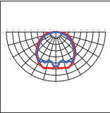
DN = Ottica in policarbonato diffondente trasparente Transparent diffusing polycarbonate optic
