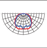
DM = Ottica in policarbonato diffondente opale Opal diffusing polycarbonate optic
