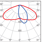
DF = Ottica stradale Classe M larghezza carreggiata < altezza palo Road optic Class M larghezza carreggiata < pole height
