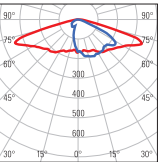
DD = Ottica stradale Classe M3-M4 - Type III (medium) larghezza carreggiata > altezza palo Road optic Class M3-M4 - Type III (medium) larghezza carreggiata > pole height
