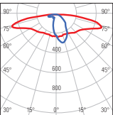
DB = Ottica stradale Classe M3-M4 larghezza carreggiata ≤ altezza palo Road optic Class M3-M4 carriageway width ≤ pole height for high pole spacing
