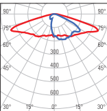
DD = Ottica stradale Classe M3-M4 - Type III (medium) larghezza carreggiata > altezza palo Road optic Class M3-M4 - Type III (medium) carriageway width > pole height
