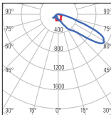
TC = Ottica centrale controflusso Central optic for counterflow
