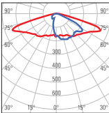
DD = Ottica stradale Classe M3-M4 - Type III (medium) larghezza carreggiata > altezza palo Road optic Class M3-M4 - Type III (medium) larghezza carreggiata > pole height
